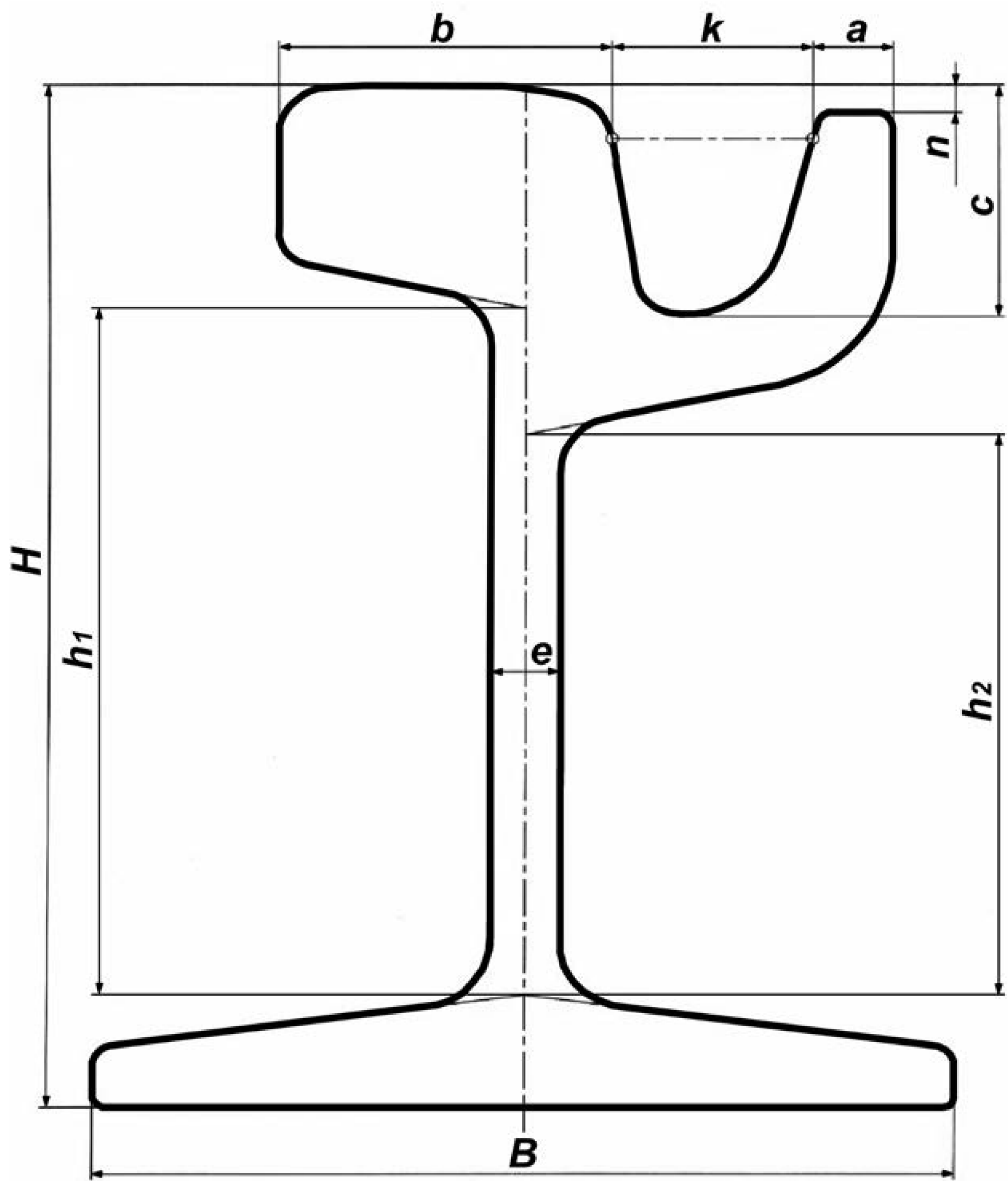
Рисунок 1 — Основные размеры поперечного сечения желобчатых рельсов
